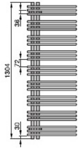
Widok boczny: jednowarstwowa
