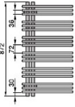
Widok z przodu: wersja prawa
