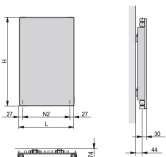
Zasilanie wodne - model VZAD (pionowy dwuwarstwowy)
