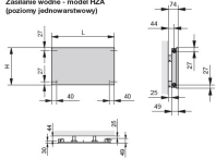
Zasilanie wodne - model H2LA (poziomy jednowarstwowy z lamelami)
