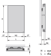
Zasilanie wodne - model VZAD (pionowy dwuwarstwowy)
