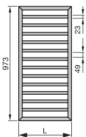
Widok z przodu, SUB-100
