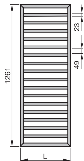
Widok z przodu, SUB-130
