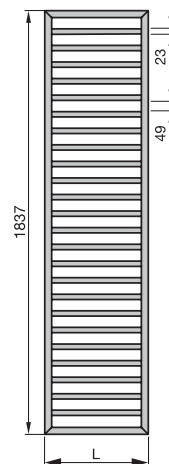
Widok z przodu, SUB-180
