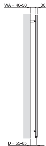
Widok z boku, SUB-180
