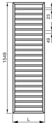
Widok z przodu, SUB-150
