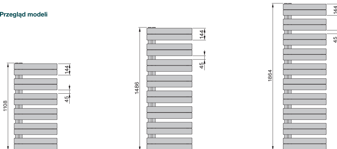
Widok z przodu - wersja wodna
