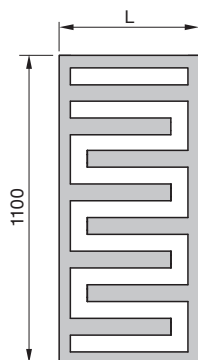
Widok z przodu TET-110-050
