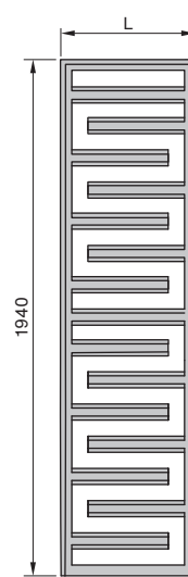
Widok z przodu TET-190-050
