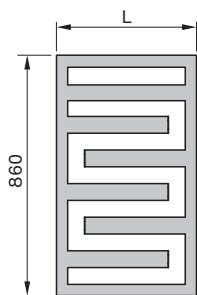
Widok z przodu TET-090-050
