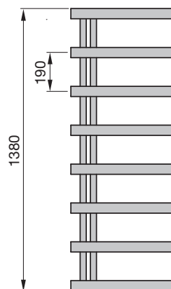
Widok z przodu CHZ-140-050
