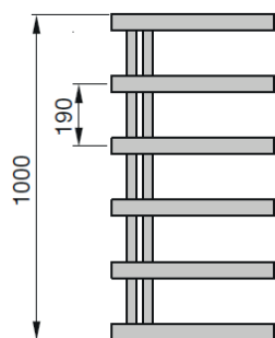
Widok z przodu CHZ-100-050
