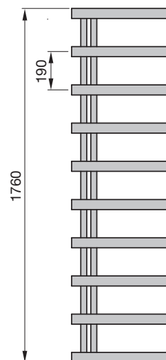
Widok z przodu CHZ-180-050
